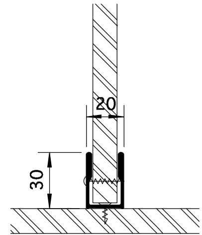
raccord de paroi intermédiaire paroi frontale en aluminium
